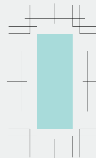
パッド印刷範囲 W15×H40mm
