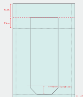
【袋展開図】
